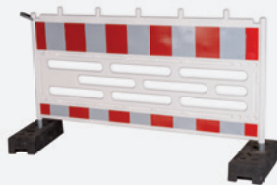
10024.3 Płotek zabezpieczający plastikowy, z mocowaniem lamp, folia RA2 ciemniejszy / Plastic barrier fence with lamp holder Foil RA1, dark
